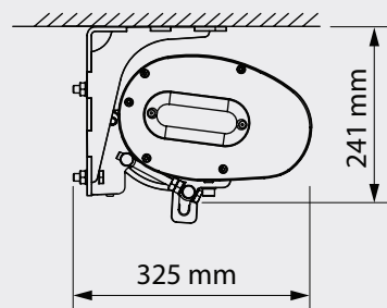
vägg installation
