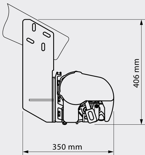
installation mot takstol
