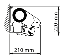
vägg installation
