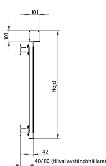
Snäppskena
