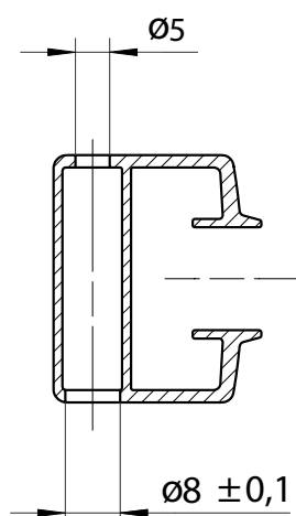
Sidoskena inkl. storlek på borrhålen
