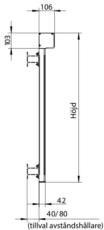
Snäppskena
