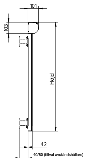
Snäppskena
