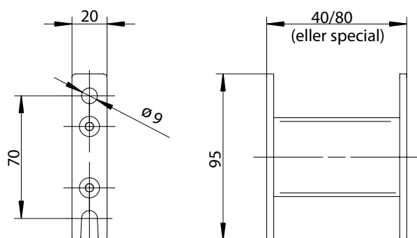
Avståndshållare (tillval)
