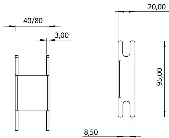
Avståndshållare Basic (tillval)
